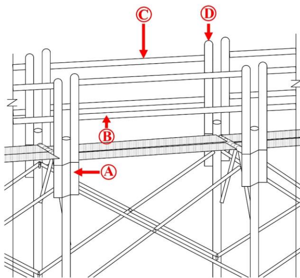
圖：先行扶手框構造示意圖
